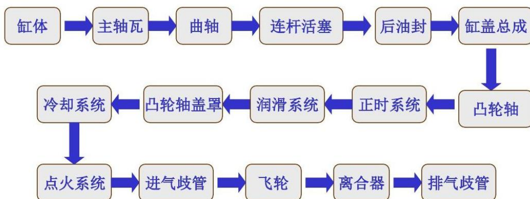
图 3-3 柴油发动机装配工艺流程图
